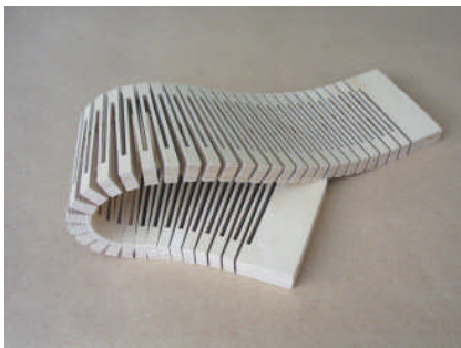
Holzpreis Schweiz – Prix Lignum 2009: Hauptpreis Region Nord Einschnittverfahren „Dukta“ zur dreidimensionalen Verformung von Holzwerkstoffplatten. Idee, Konzept, Gestaltung: Serge Lunin, Christian Kuhn, Zürich
